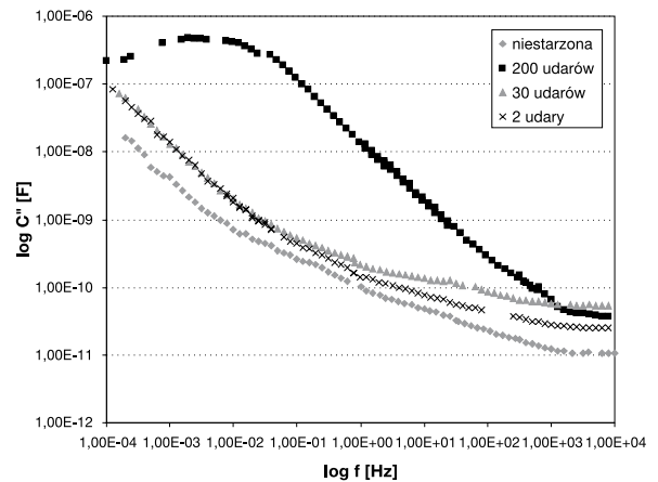
Rys. 5. Widma częstotliwościowe składowej urojonej pojemności zespolonej C''
