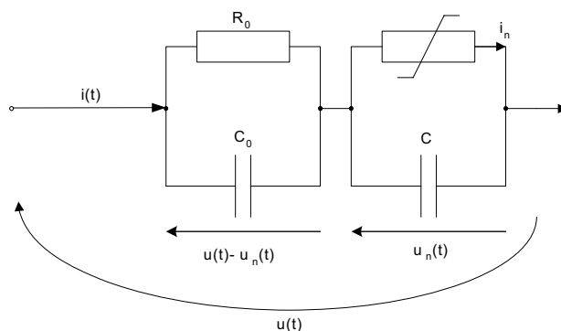
Rys.1. Model analityczny warystora ZnO
